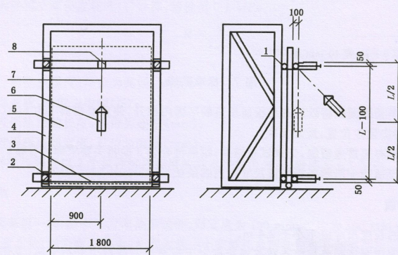
a) 正立面示意图
