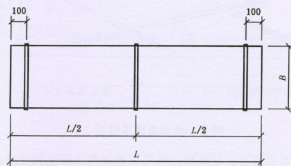
图3 宽度测量位置
