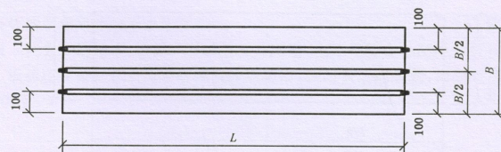
图2 长度测量位置
