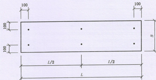
图4 厚度测量位置
