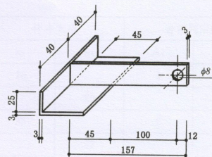
图 9 钢板吊挂件
